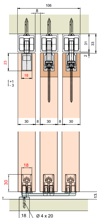
Conjunto 3 PORTAS Espessura fixa 30mm
