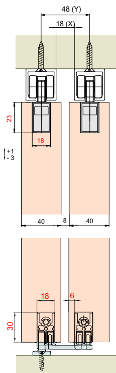
Conjunto 2 PORTAS Espessura flexível (Exemplo 40mm)
